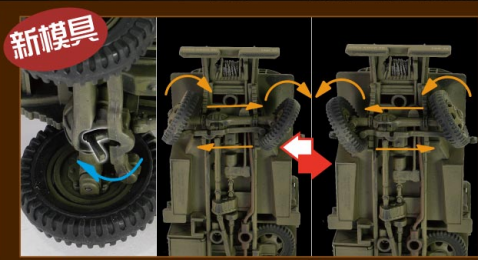
前轮卡扣锁-解锁后能随意调整车轮转向
