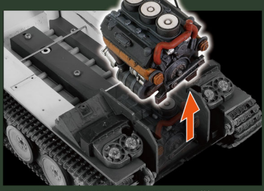
迈巴赫HL-210 P45发动机及散热器细节
